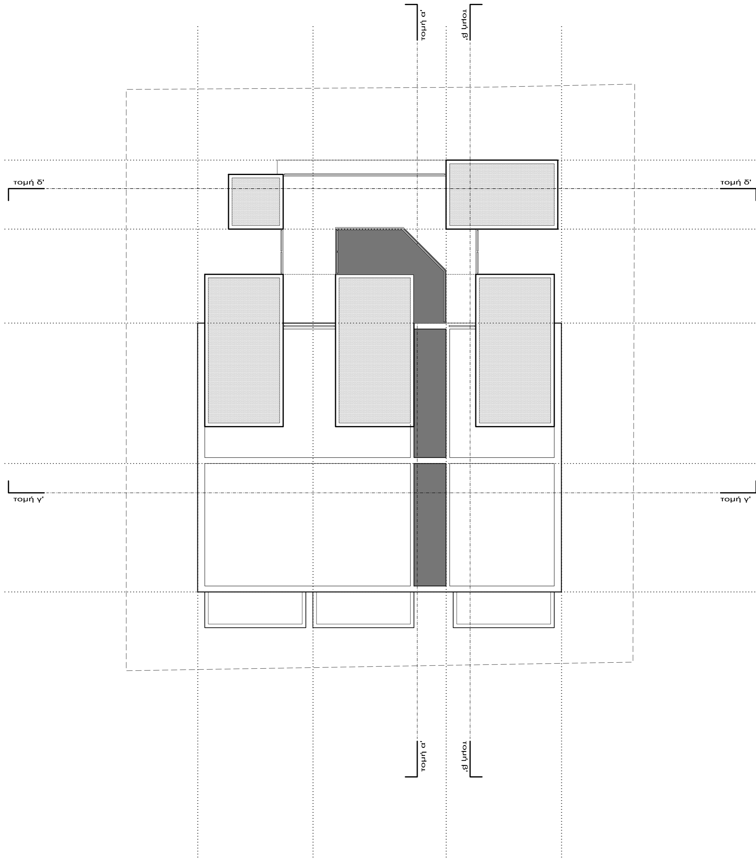
κάτοψη οροφών_1:100
