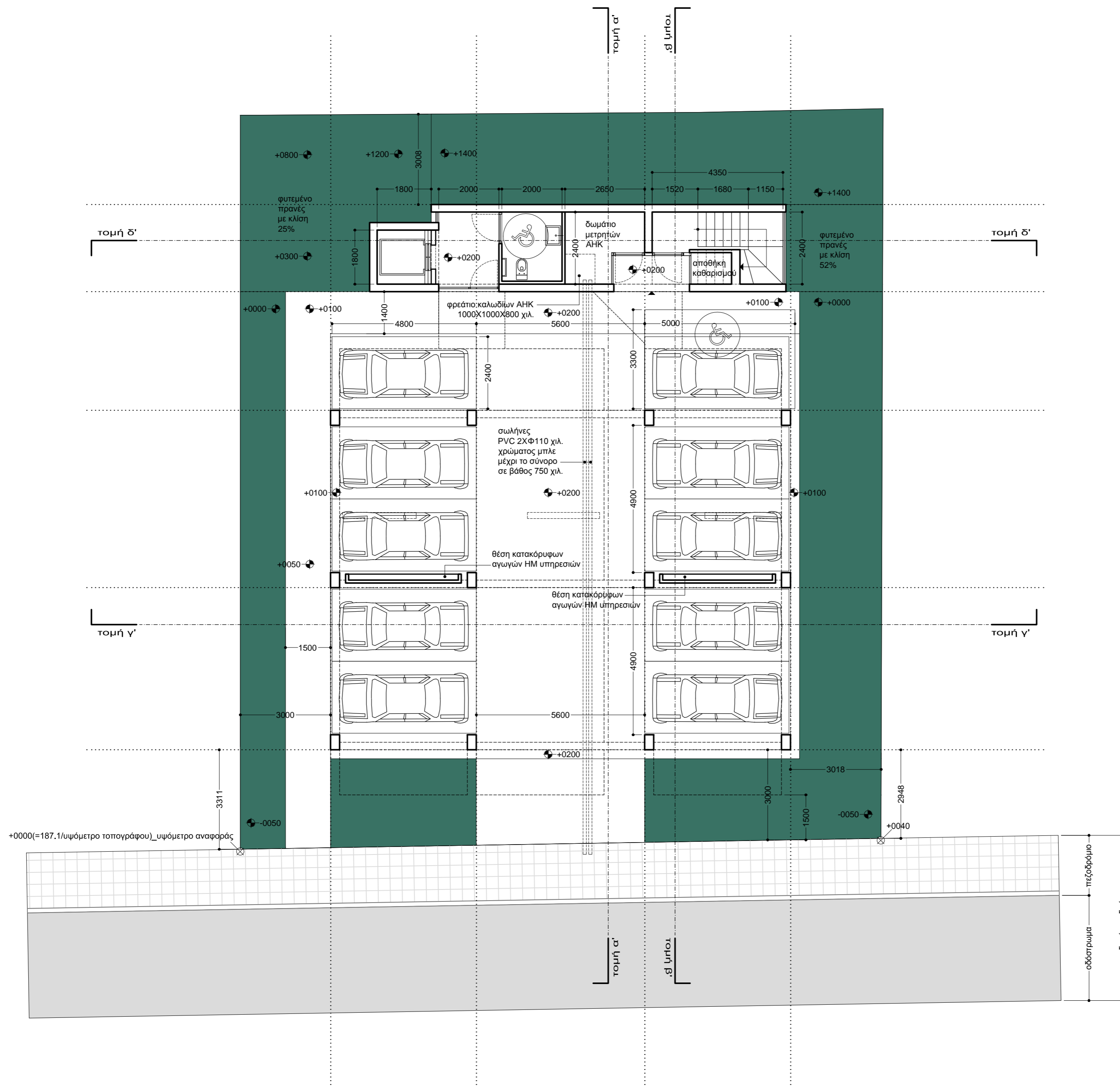
κάτοψη ισογείου_1:100
