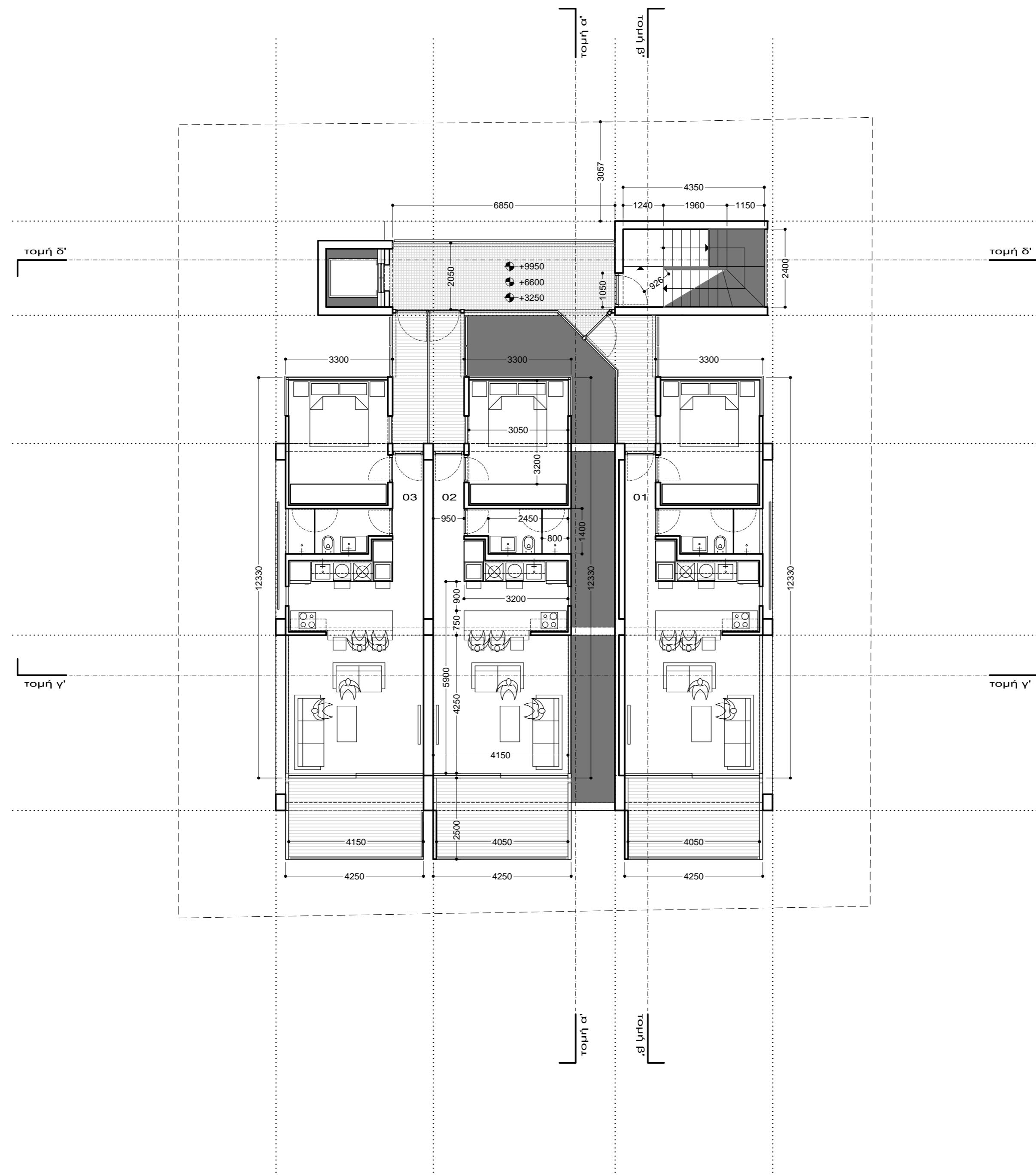
κάτοψη τυπικού 1-2-3ου ορόφου_1:100
