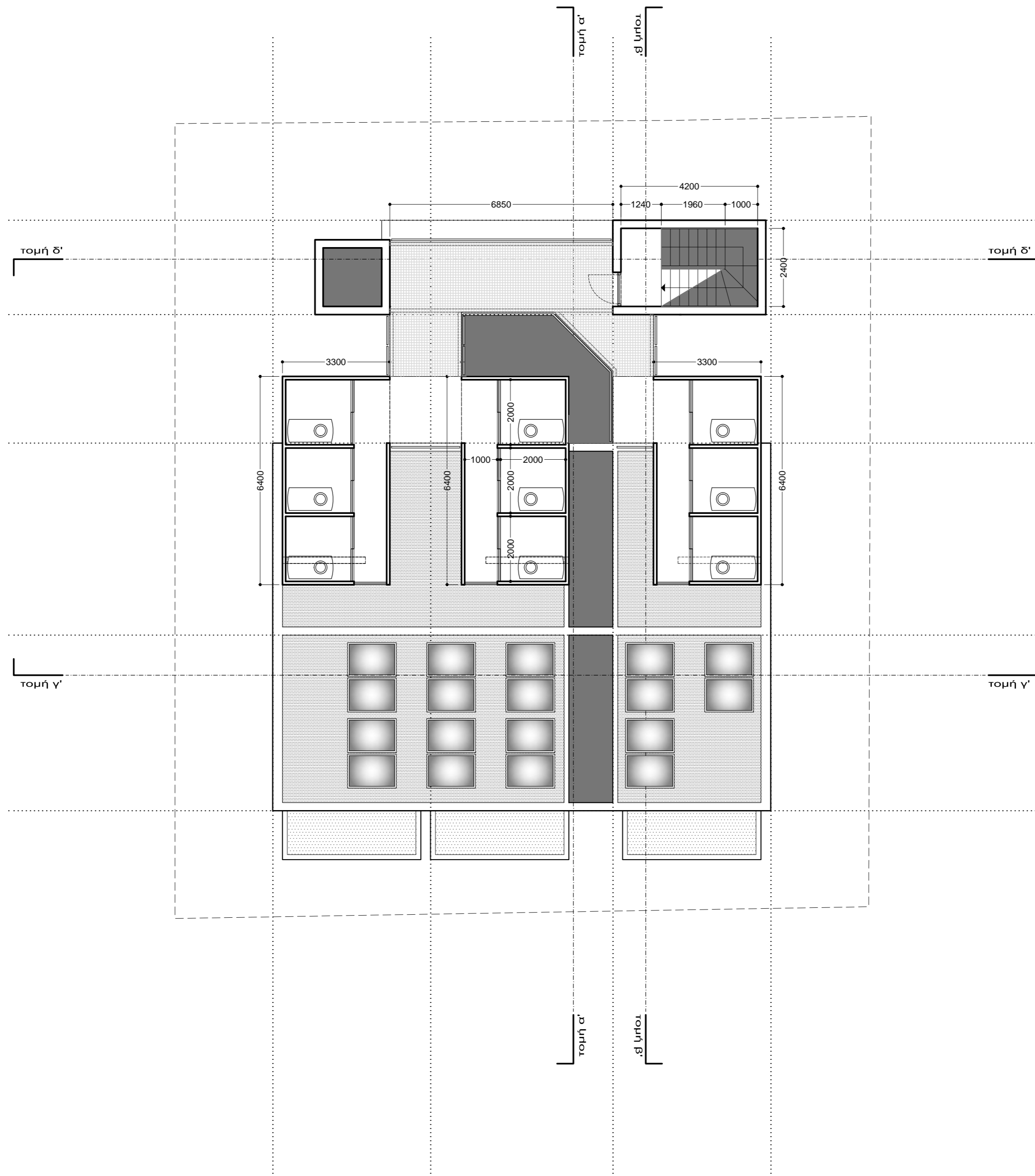
κάτοψη δώματος_1:100
