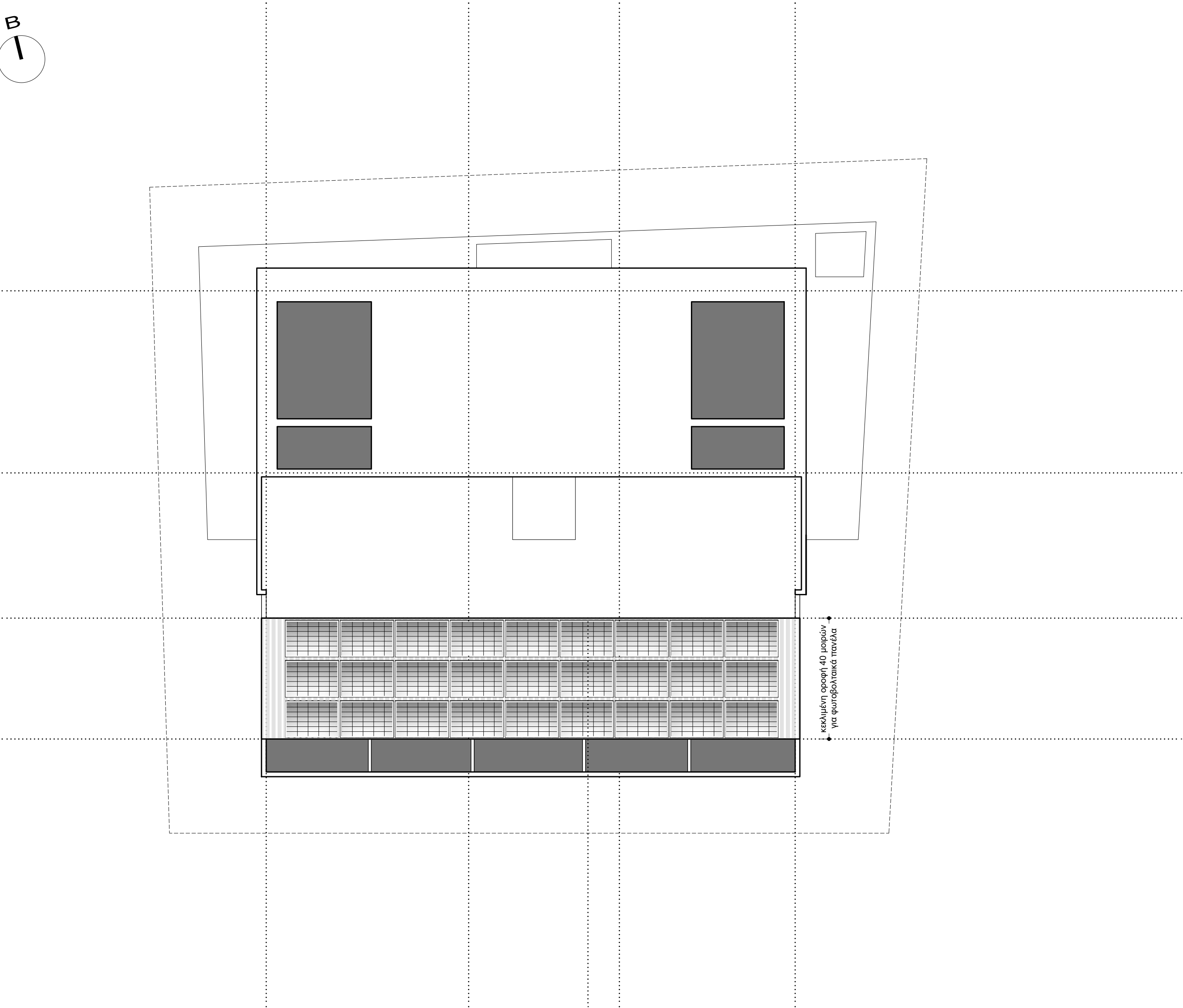
κάτοψη οροφών_1:100
