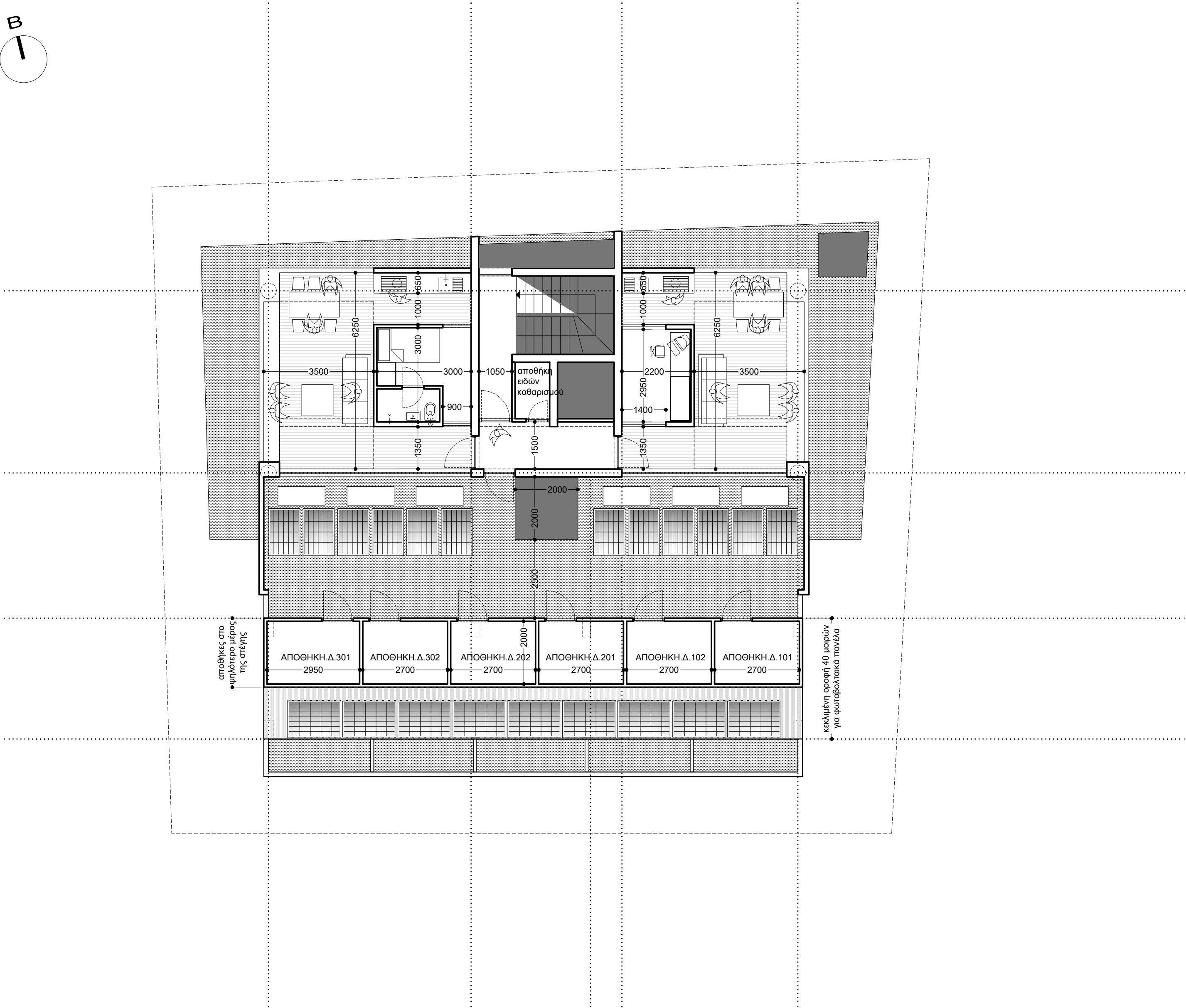
κάτοψη δωματίων_1:100
