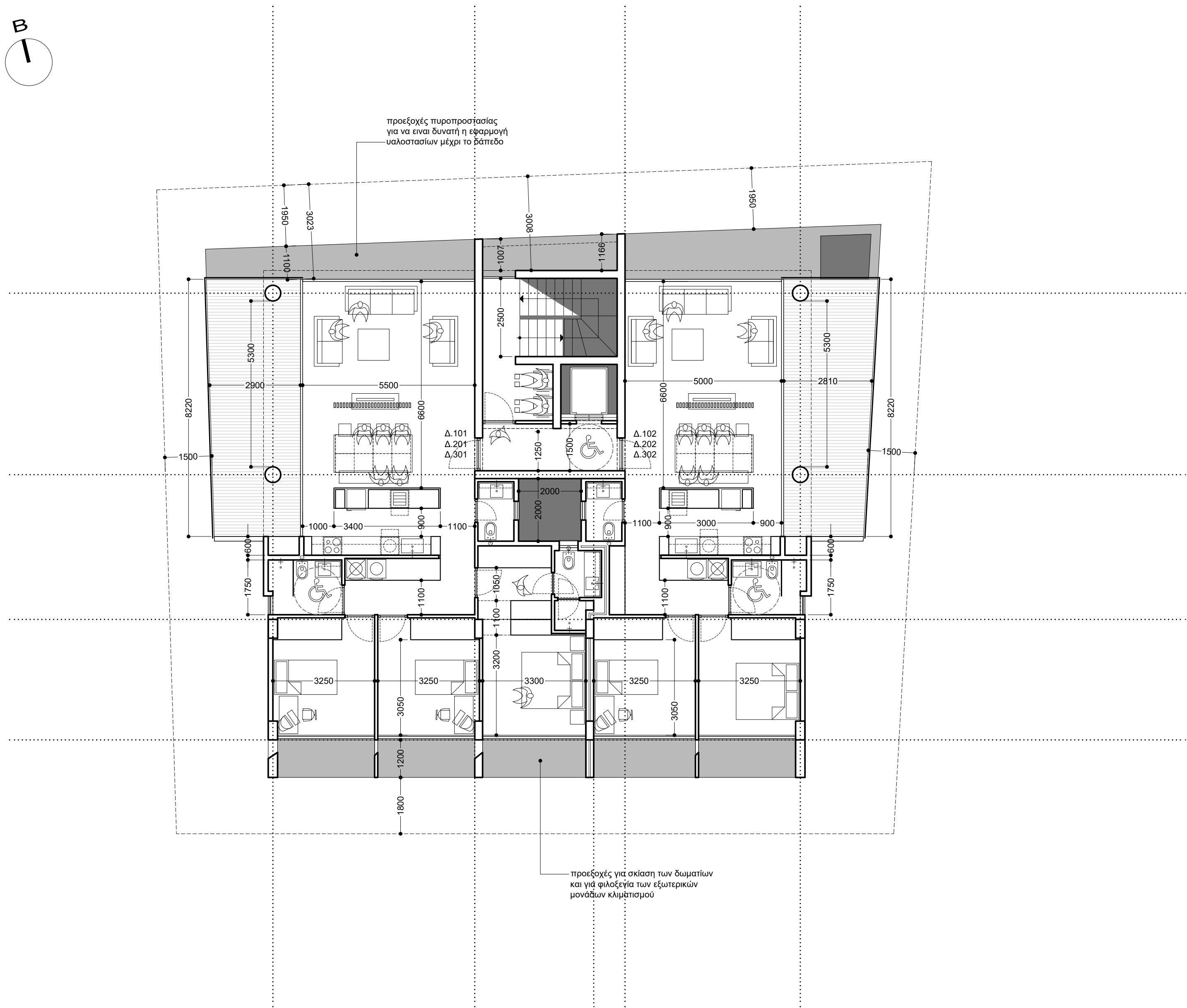
κάτοψη τυπικού ορόφου (1-2-3ος)_1:100
