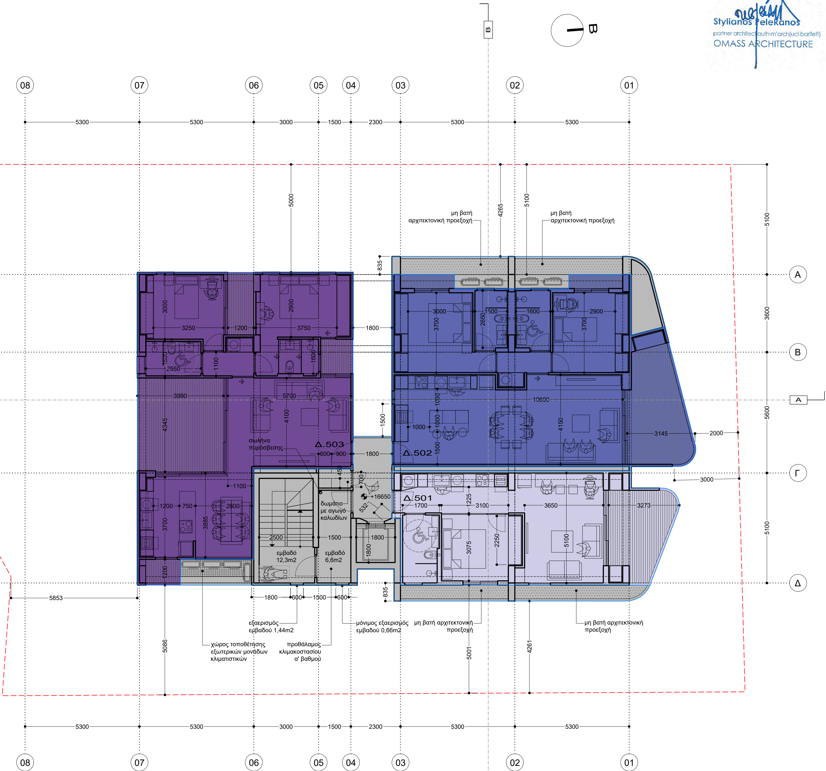
κάτοψη 5ου ορόφου_1:100
