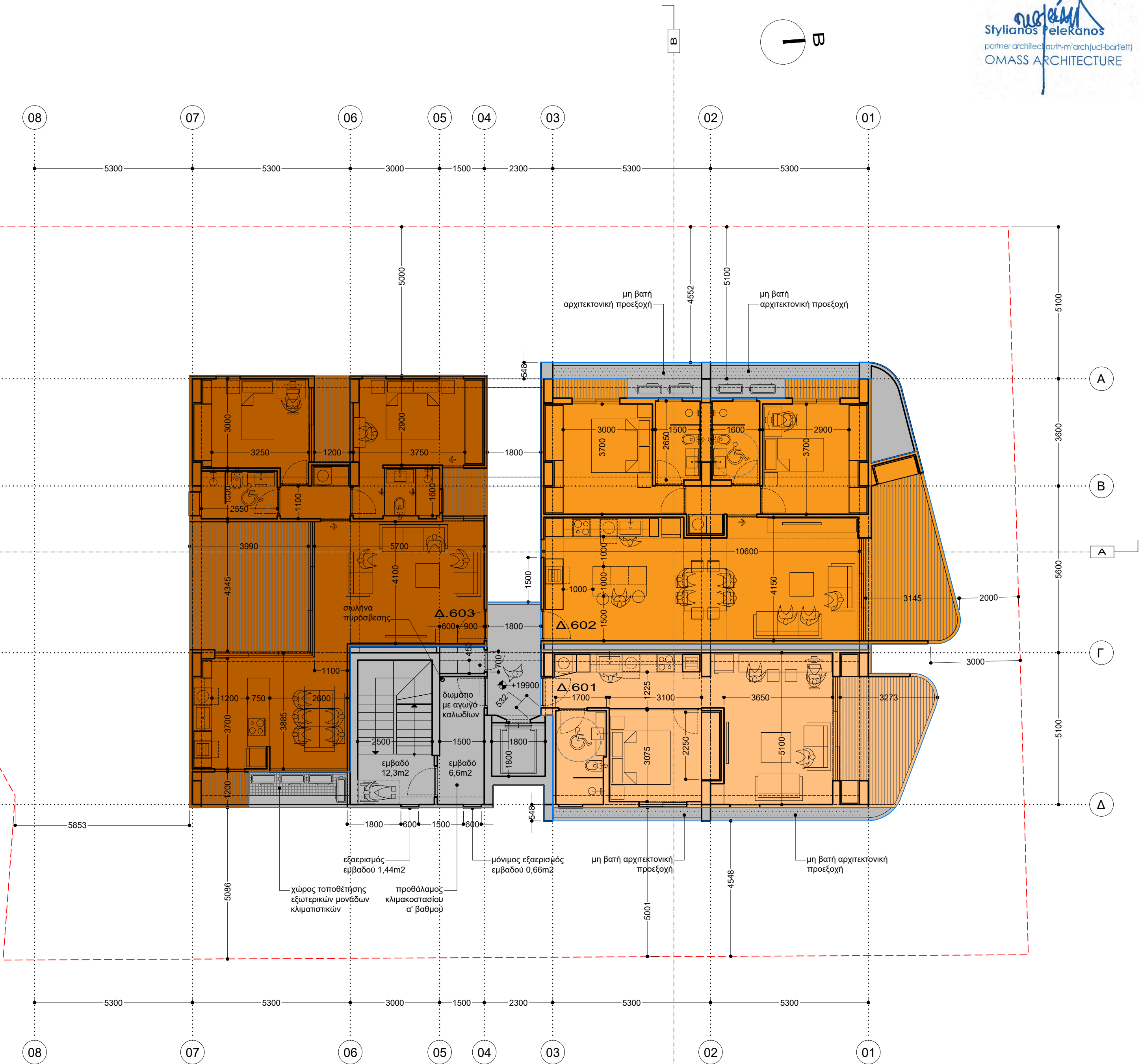
κάτοψη 6ου ορόφου_1:100
