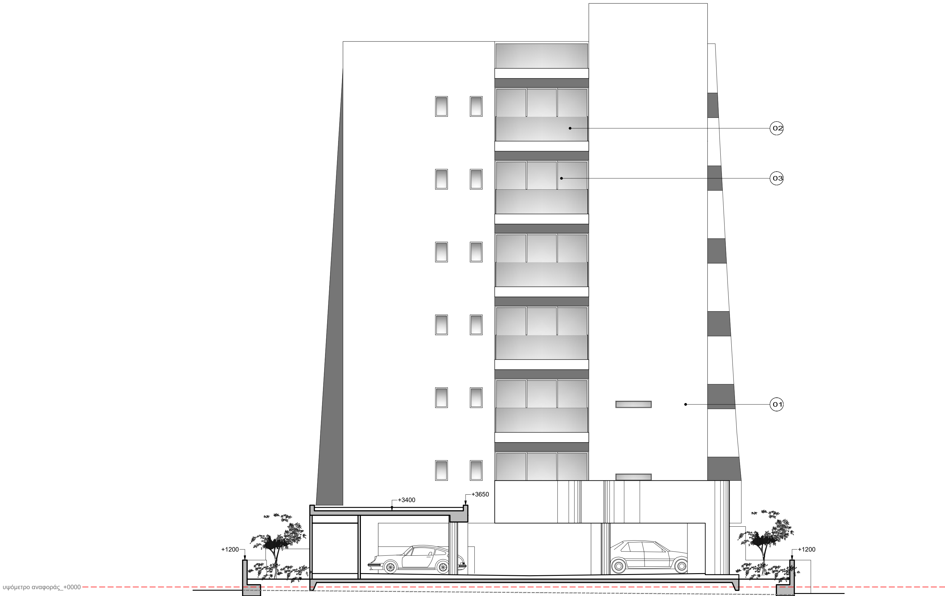
νότια όψη_1:100
