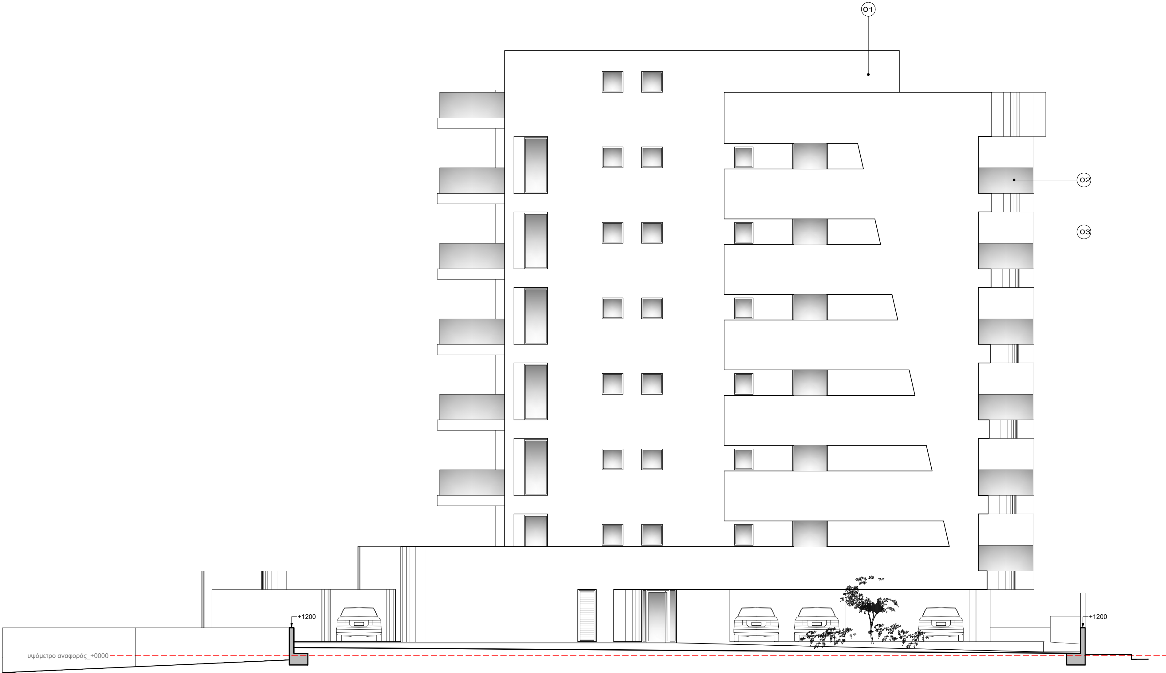
ανατολική όψη_1:100
