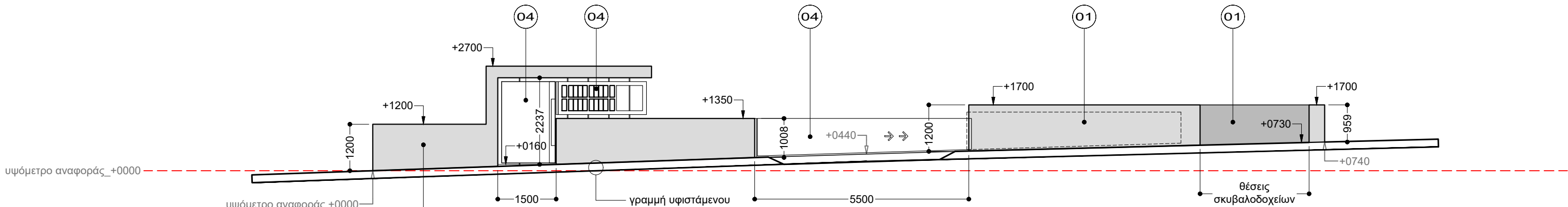
περίφραξη βόρειας όψης_1:100
